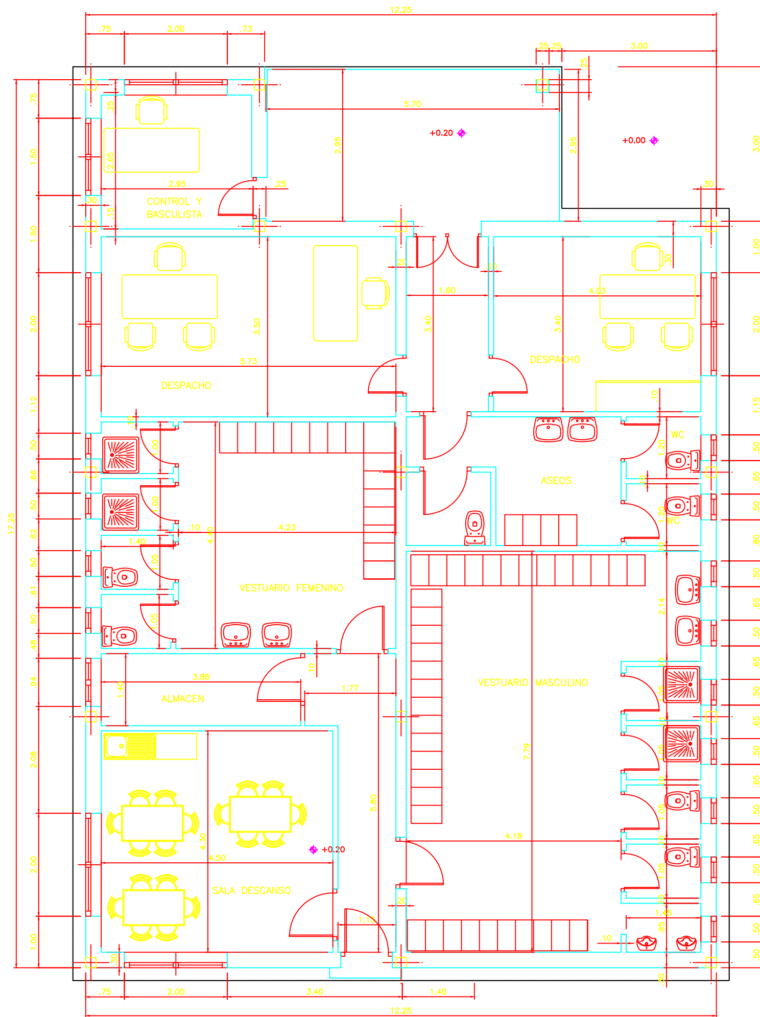
PLANTA ACOTADA ESCALA: 1/50
